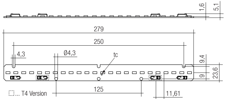
LLE G4 24x280mm 1250lm ADV
