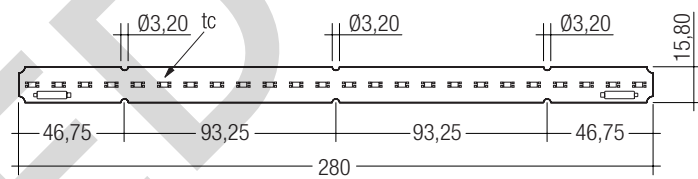
LLE G3 16x280mm 1250lm ADV
