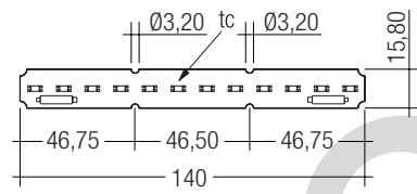
LLE G3 16x140mm 650lm ADV
